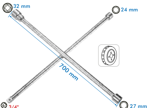
CLÉ EN CROIX 3/4"
